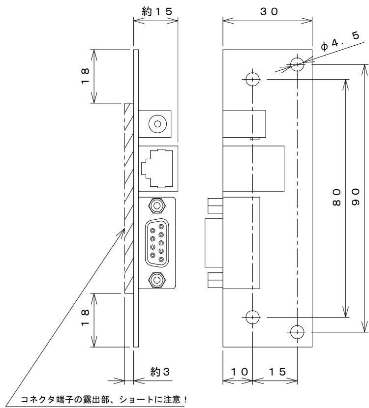
中継基板
